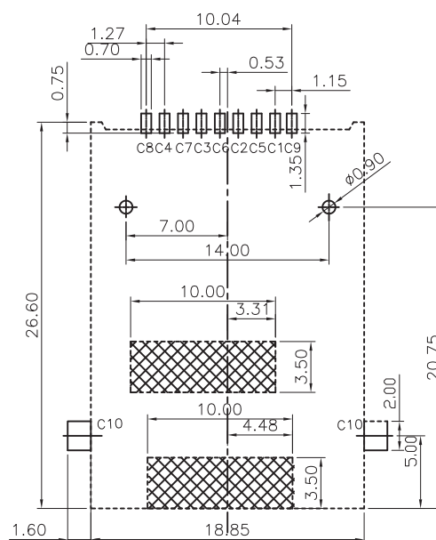
P.C.B. LAYOUT
