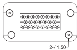
KEYING PCB
