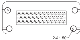
KEYING PCB
