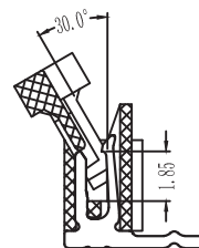
A-A
