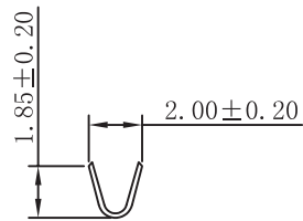
SEC A-A
